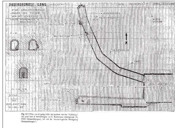
Situeringsschema van de ondergrondse gang onder het podium en in de tuin van het Volkshuis, getekend door Dirk Roelandt.
